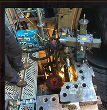
ÉLECTROÉROSION - DESTRUCTION ÉCROUS EDM - destruction of nuts
