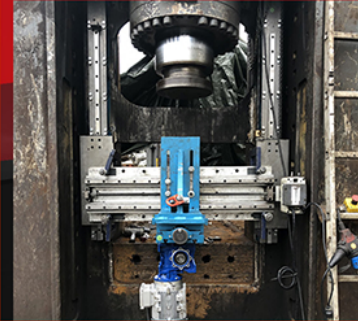
FRAISAGE LOGEMENT LAME APRÈS RECHARGEMENT SUR CISAILLE / Blade housing milling after reloading on a shear
