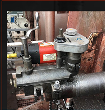
FRAISAGE DE 2 RAINURES SUR ARBRE Slot milling key on shaft
